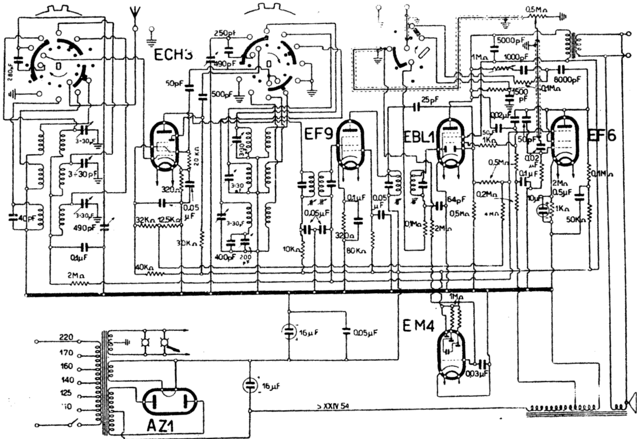
PHILIPS RADIO - MOD. « 478 »
